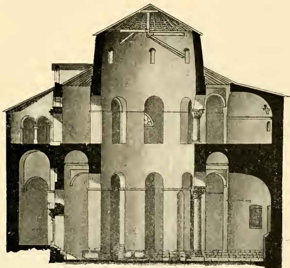
Fig. 299 — Rotonda di San Donato a Zara. Spaccato (a. Stz)
